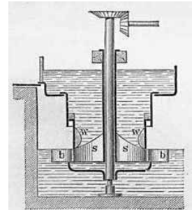
Sección de una turbina de agua
